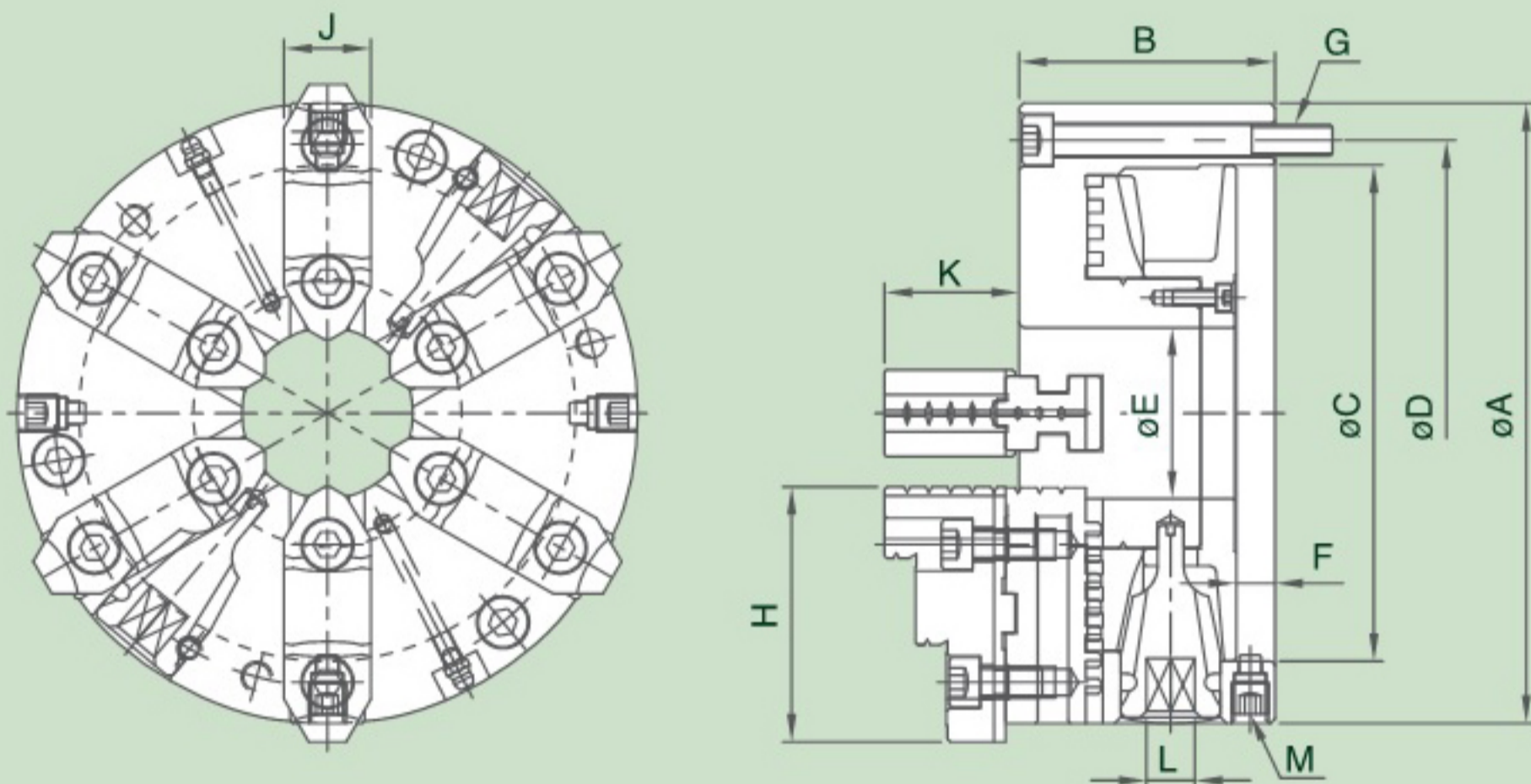
尺寸圖 » Dimensions
