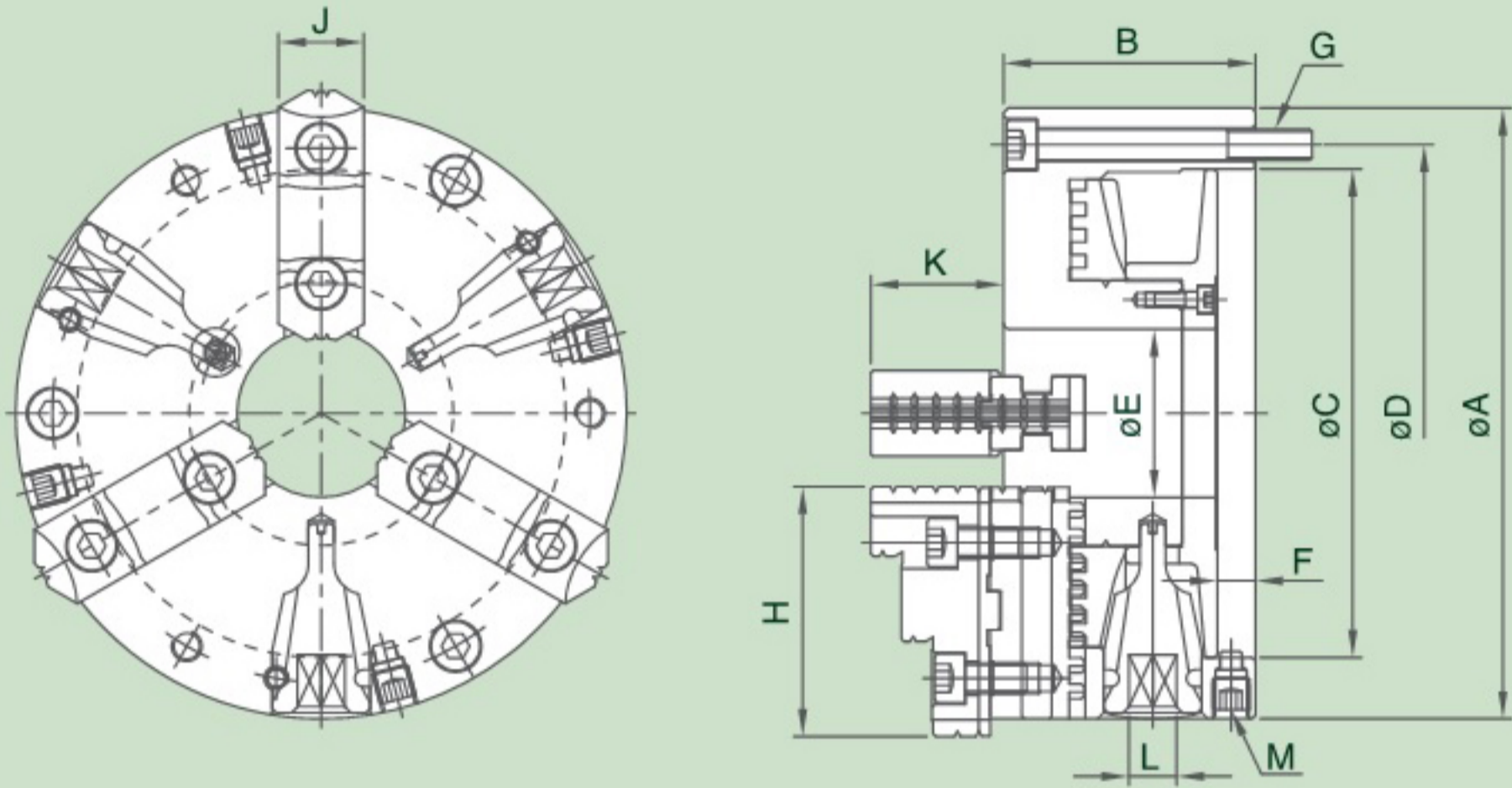
尺寸圖 » Dimensions
